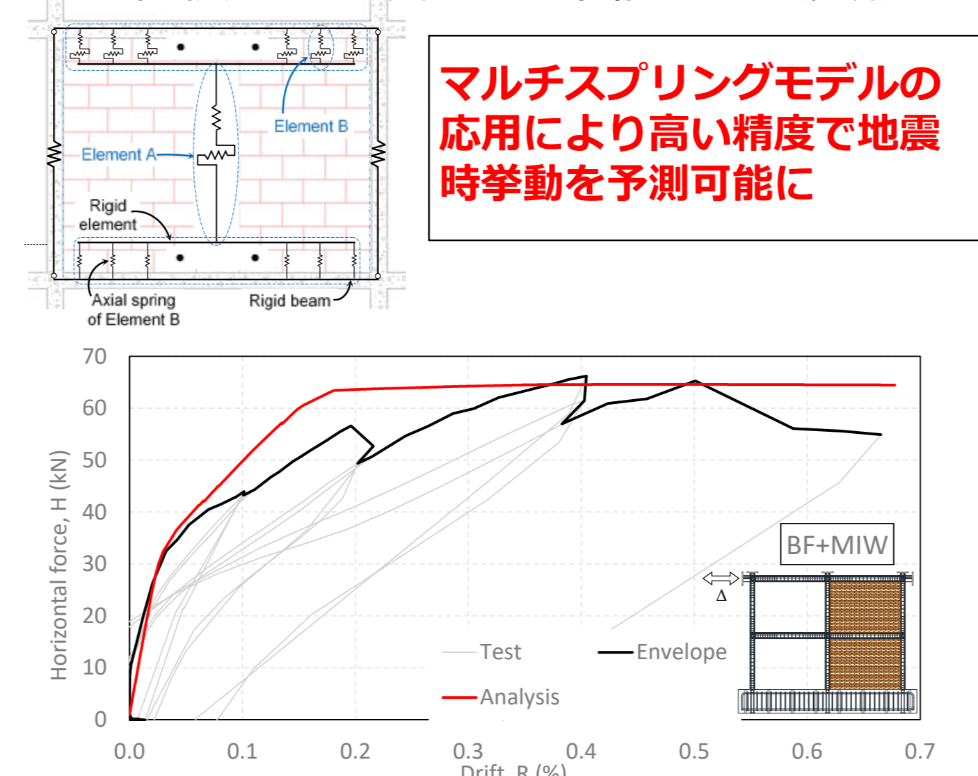
モデル化のコンセプトと実験結果との比較
