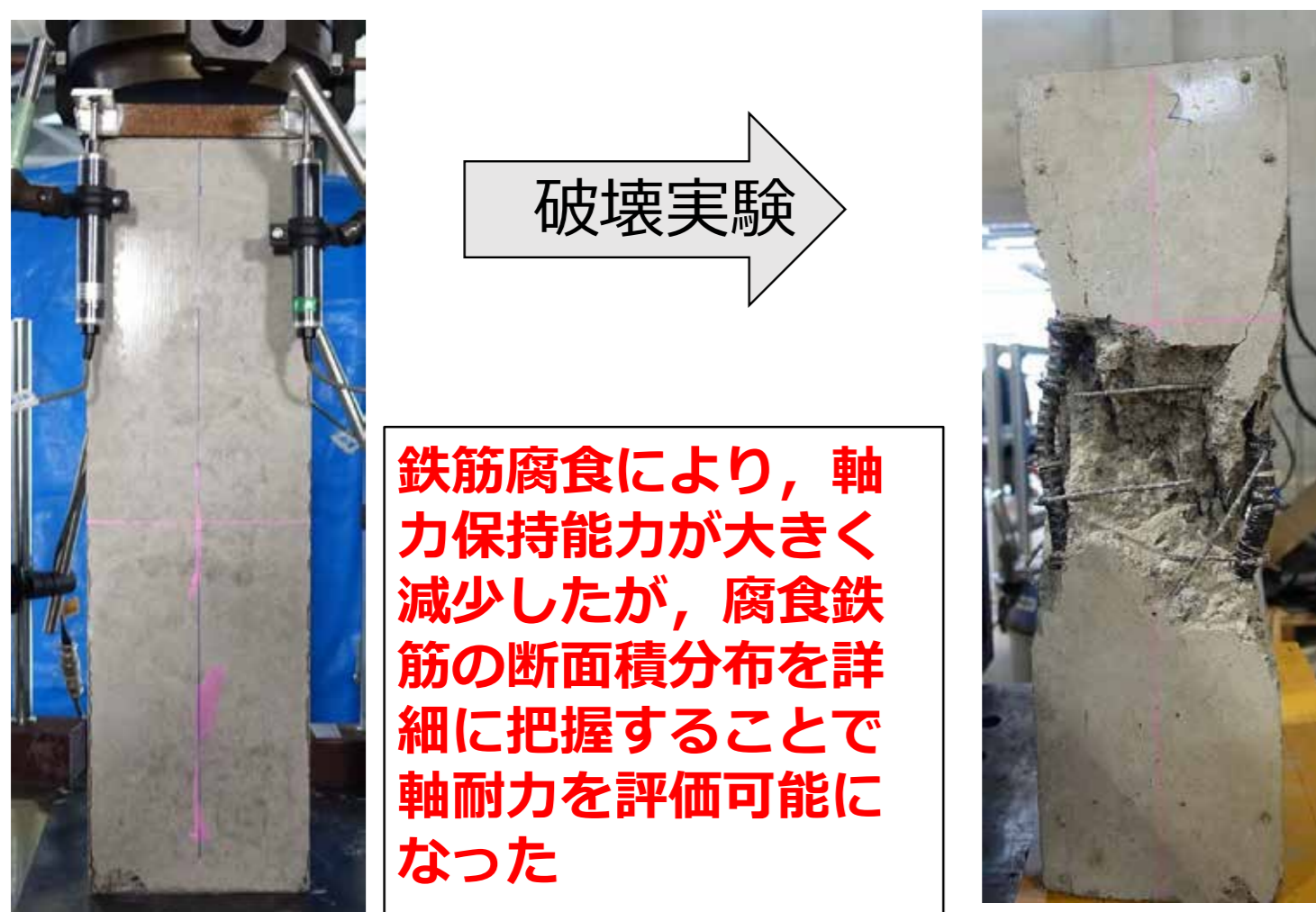
破壊実験による軸耐力評価
