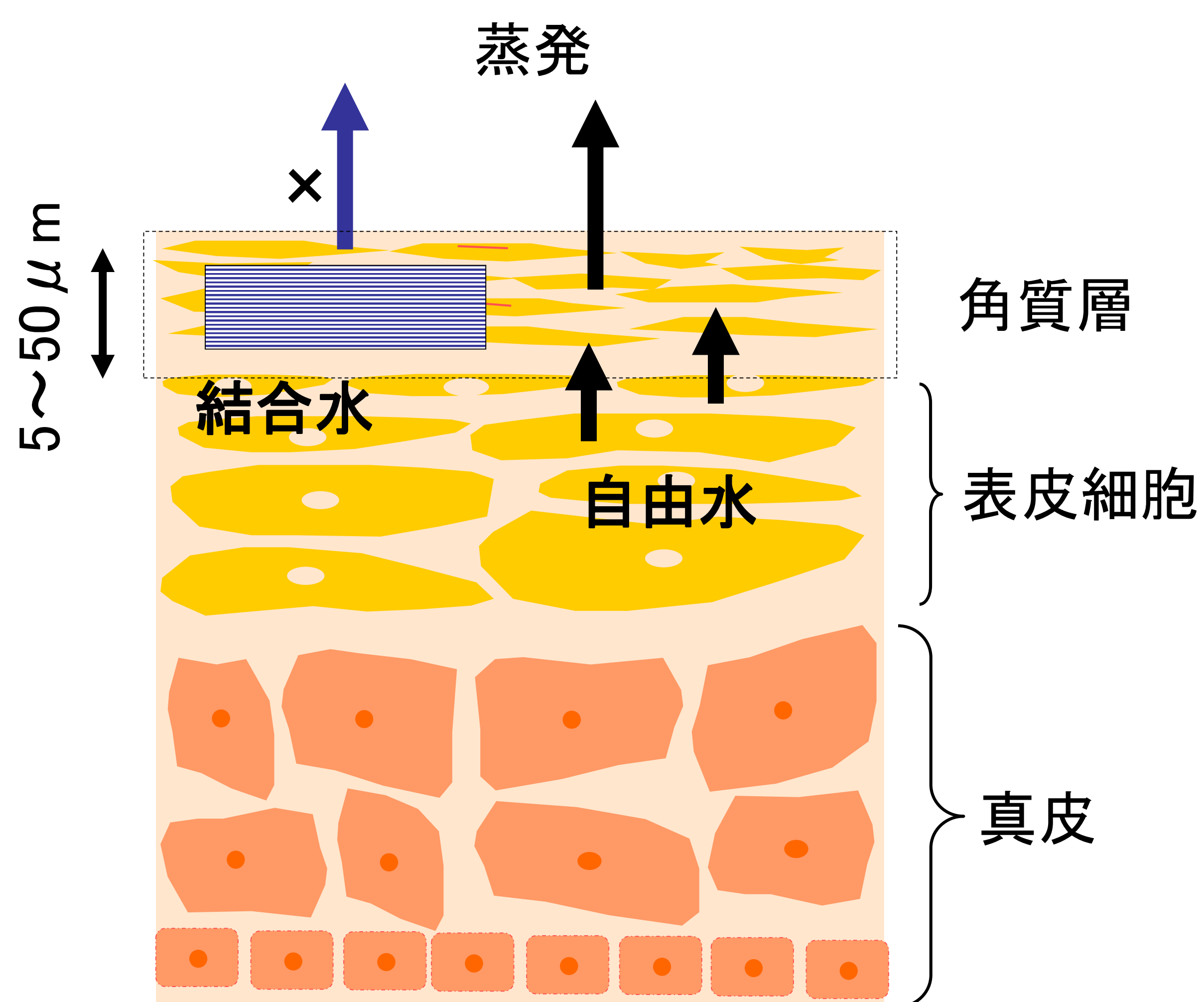
図1. 皮膚と水分蒸発の模式図
