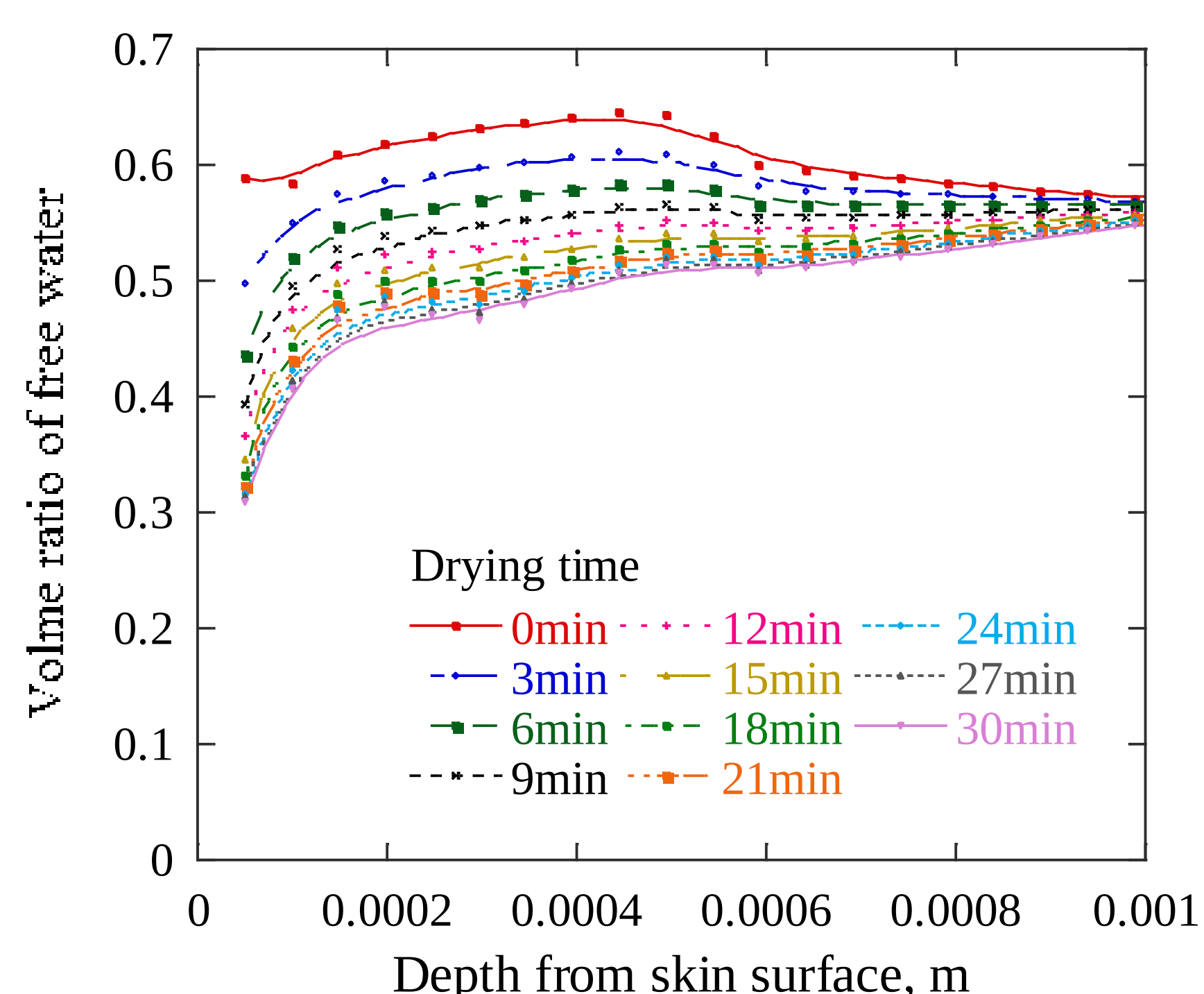
図3. 蒸発過程の皮膚内自由水分分布
