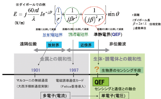
準静電界と他の電磁界との違い
