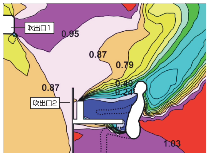
室内換気効率（空気齢）のCFD解析結果
