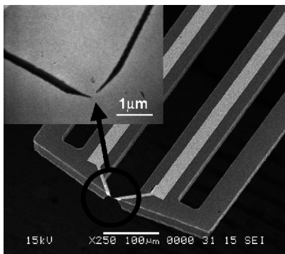
太さ0.1μmの可動ツインプローブ
