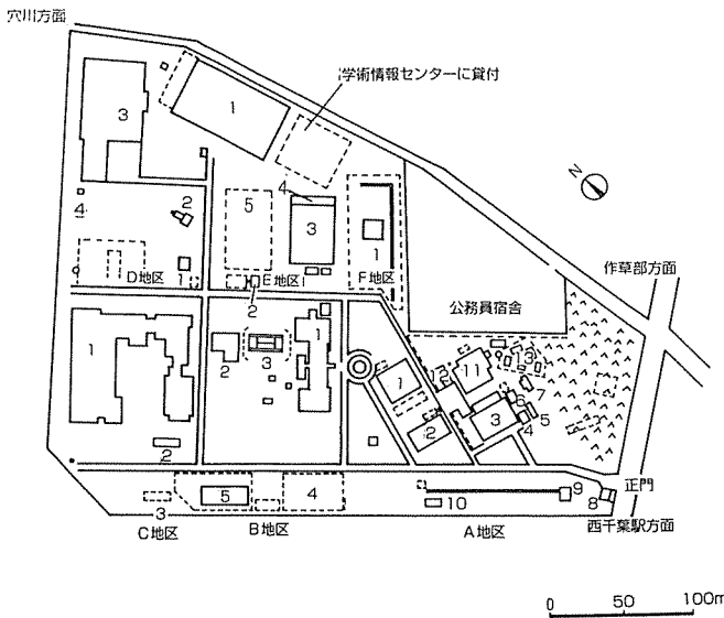
東京大学生産技術研究所千葉実験所 配置図
