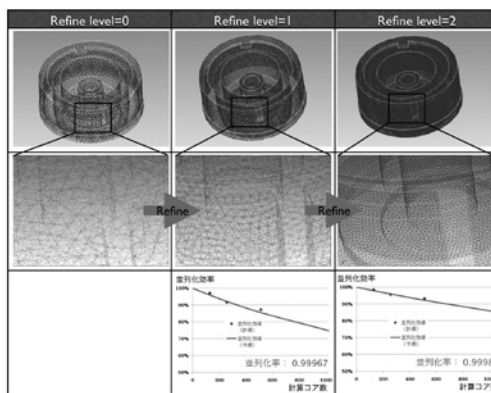
図 1：階層化メッシュの生成例と解析時並列化効率
