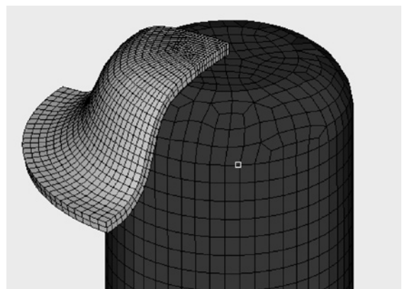
図2 プレス加工の接触解析例
