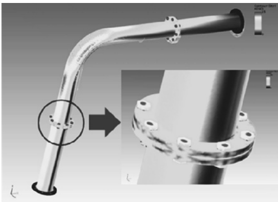
図1 アセンブリ構造の線形静解析例
