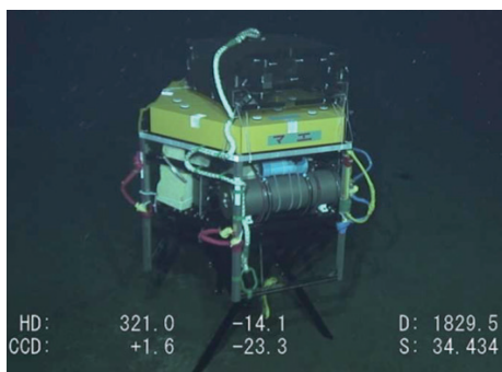
海底ステーション Underwater station
