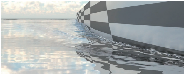
船体まわりの乱流境界層と造波の数値シミュレーション （画像提供：一般財団法人日本造船技術センター） Numerical simulation of hull boundary layer and wave resistance (Courtesy of Shipbuilding Research Centre of Japan)
