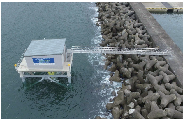
日本で初めて系統に連系した波力発電所 (2016年9月岩手県久慈市に設置) : 最大出力43 kW The Kuji Wave Power Plant (rated output 43 kW), Japan's first grid connected wave power generator
