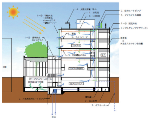
理想の教育棟ZEBのAI制御事例 (2011) 全キャンパス平均比 ▲67%省エネルギー Komaba Center for Educational Excellence ▲ 67% energy saving
