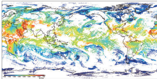
人工衛星搭載の分光計から測定した水蒸気同位体比 ( \delta D ) の分布 Distribution of water vapor \delta D observed by a satellite spectroscopic sensor
