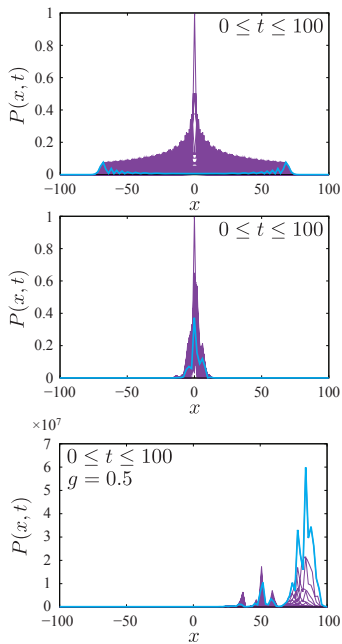
量子ウォーク (上) にランダムネス (中) と非エルミート性 (下) を入れたシミュレーション結果 Quantum walk (top) with additional randomness (mid) and non-Hermiticity (bottom)
