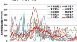
風力発電電力量の変動例
