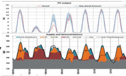
太陽光発電予測、起動停止計画、経済負荷配分シミュレーションの例
