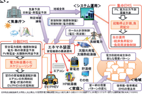
需要の電動化と集中/分散のエナジーの協調
