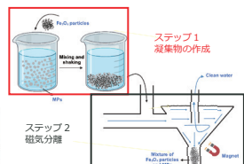
水中マイクロプラスチック (MP) の回収技術開発 磁力供用の小型サイクロン分離機によるMPの回収
