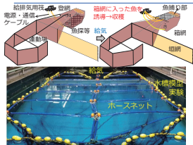
定置漁業自動魚群誘導システム 揚網作業の省力化を目指しています。
