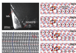
図2. \alpha\text{-Al}_2\text{O}_3 における双晶の成長挙動観察、界面原子構造、原子レベルシミュレーション
