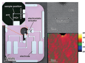
図1. 荷重負荷MEMSデバイスを用いた原子分解能TEMその場機械試験
