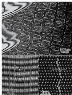
図3. らせん転位ネットワーク( \alpha\text{-Al}_2\text{O}_3 )、転位のコア構造( \alpha\text{-Al}_2\text{O}_3 )、積層欠陥構造(4H-SiC)
