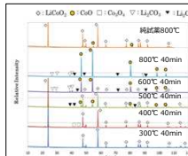
加熱後の正極材のXRDスペクトル
