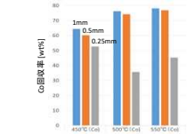
各ふるいのメッシュ幅/緩昇温加熱の違いによるCo回収率の関係
