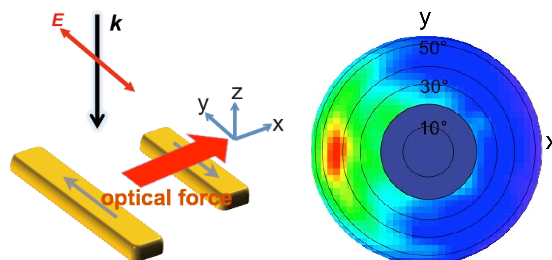
金ナノ構造による光散乱方向制御と面内放射圧
