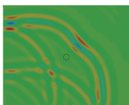
CFRP衝撃損傷のモデル化と FEM波動伝播シミュレーション
