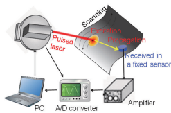
レーザー超音波可視化検査装置 (LUVI-CP, つくばテクノロジー (株))
