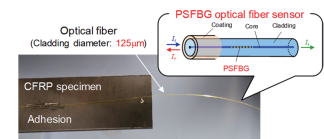
遠隔AE計測を実現する光ファイバ超音波センサ
