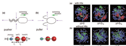
図5. 自己推進性を備えた微生物のミニマルモデルの例
