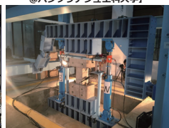
鉄筋コンクリート造架構への模擬船舶の衝突実験
