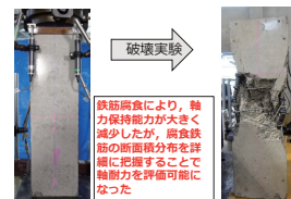
破壊実験による軸耐力評価
