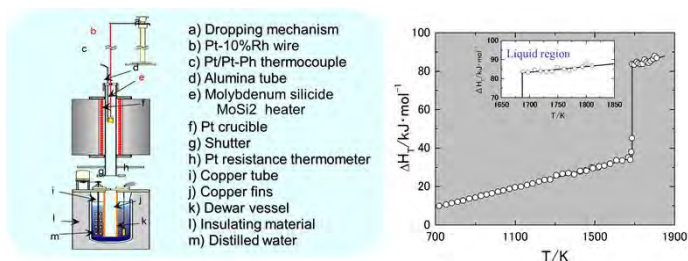
1600°Cまで使用可能な高温落下型熱量計とシリコンの高温エンタルピー
