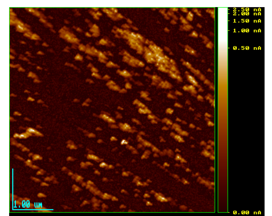
塑性変形によりGaN結晶表面に現れた導電性スポット
