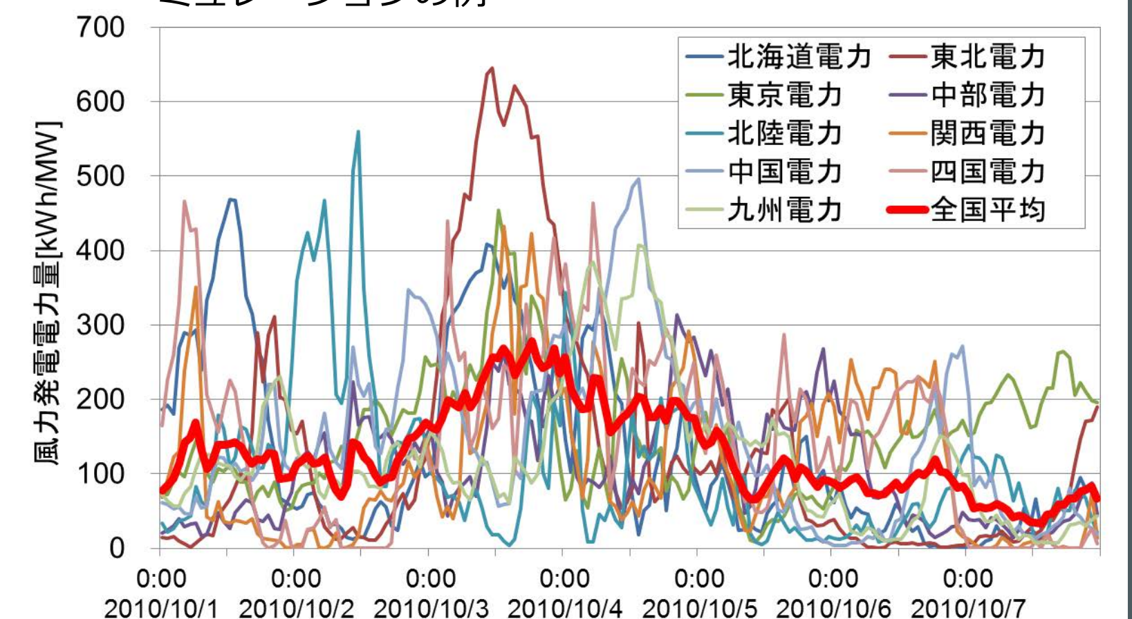
風力発電電力量の変動例
