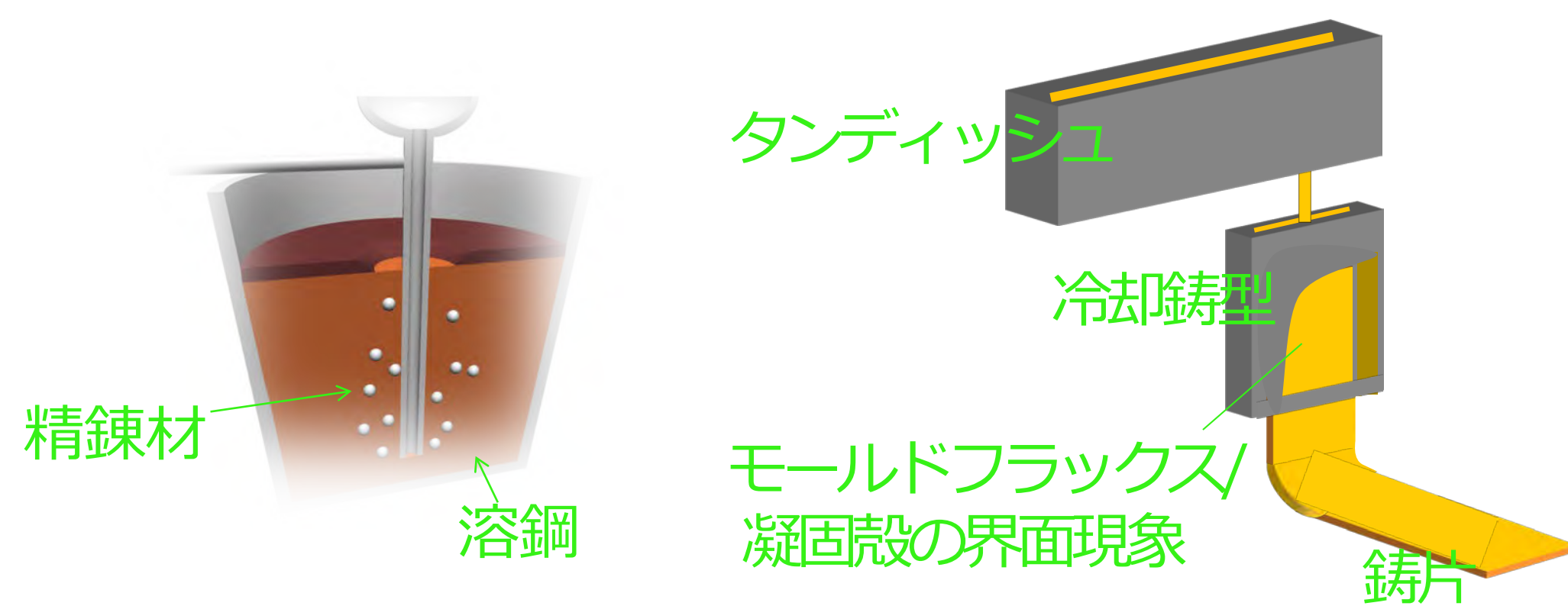
溶鋼/ 精錬材の反応制御 鑄型内の凝固組織制御
