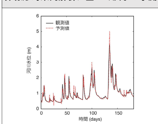
非線形時系列解析に基づく洪水の予測
