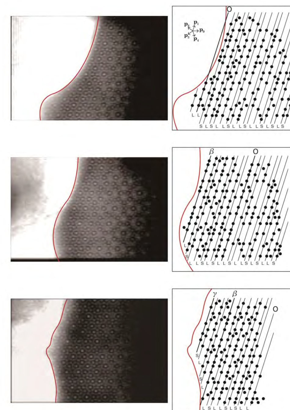
Al-Ni-Co系正10角形準結晶の成長の様子の高透過電子顕微鏡高温その場観察
