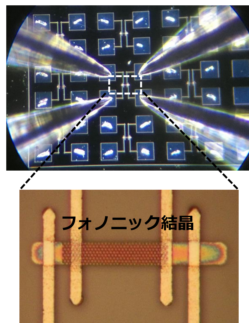
図4. 自己組織化ナノ材料を用いた安価で大面積のシリコンナノ構造を用いた環境発電デバイスとスマート社会への応用。
