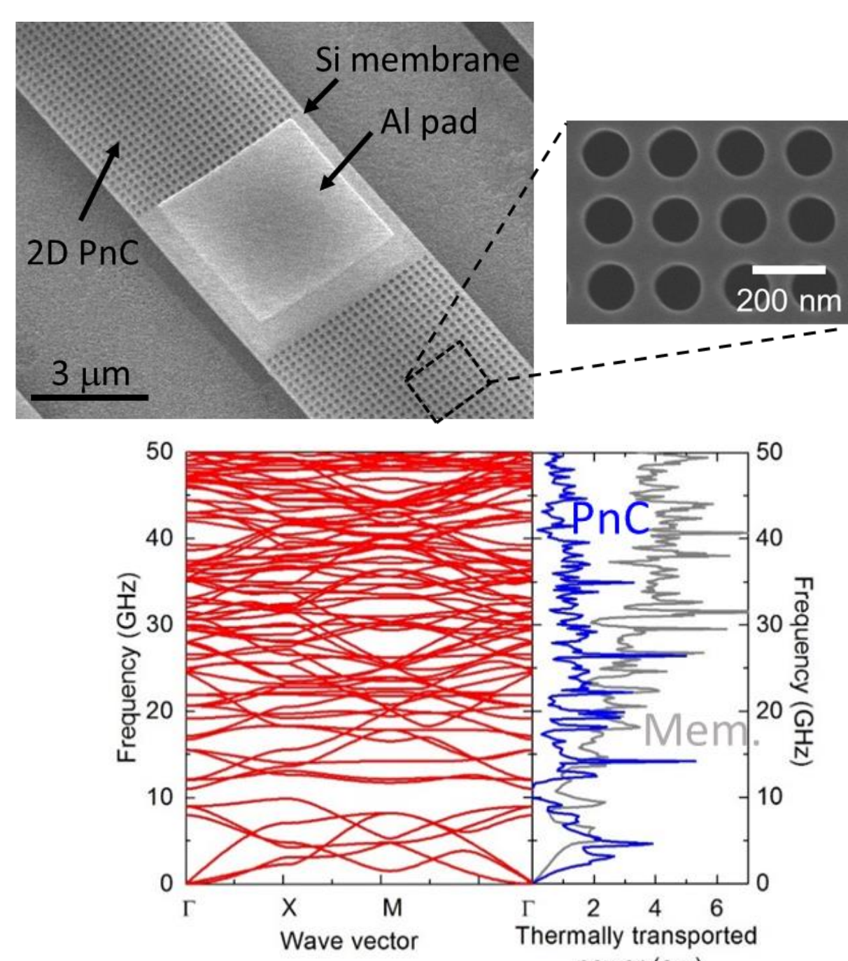
図1. フォノンニック結晶ナノ構造のSEM写真とフォノンニックバンド図および熱流束の比較。
