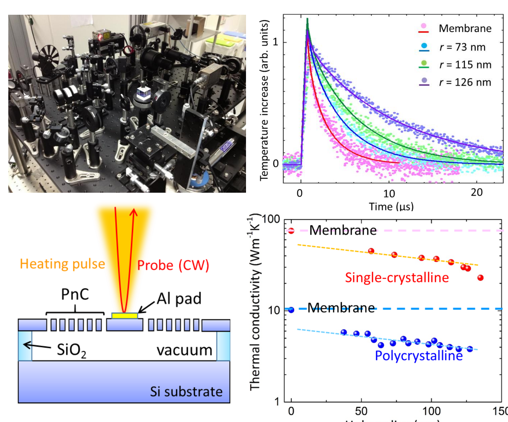
図2. マイクロサーモリフレクタンクス法と様々なフォノンニック結晶ナノ構造の熱伝導率。
