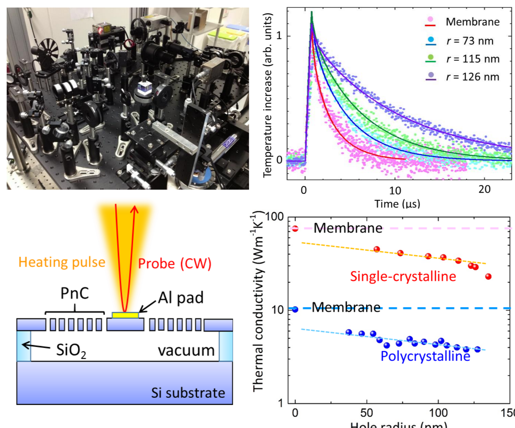
図2. マイクロサーモリフレクタンス法と様々なフォノンニック結晶ナノ構造の熱伝導率。
