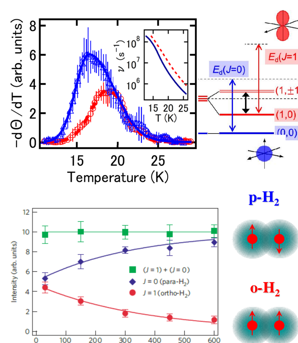
[水素の回転分光]
