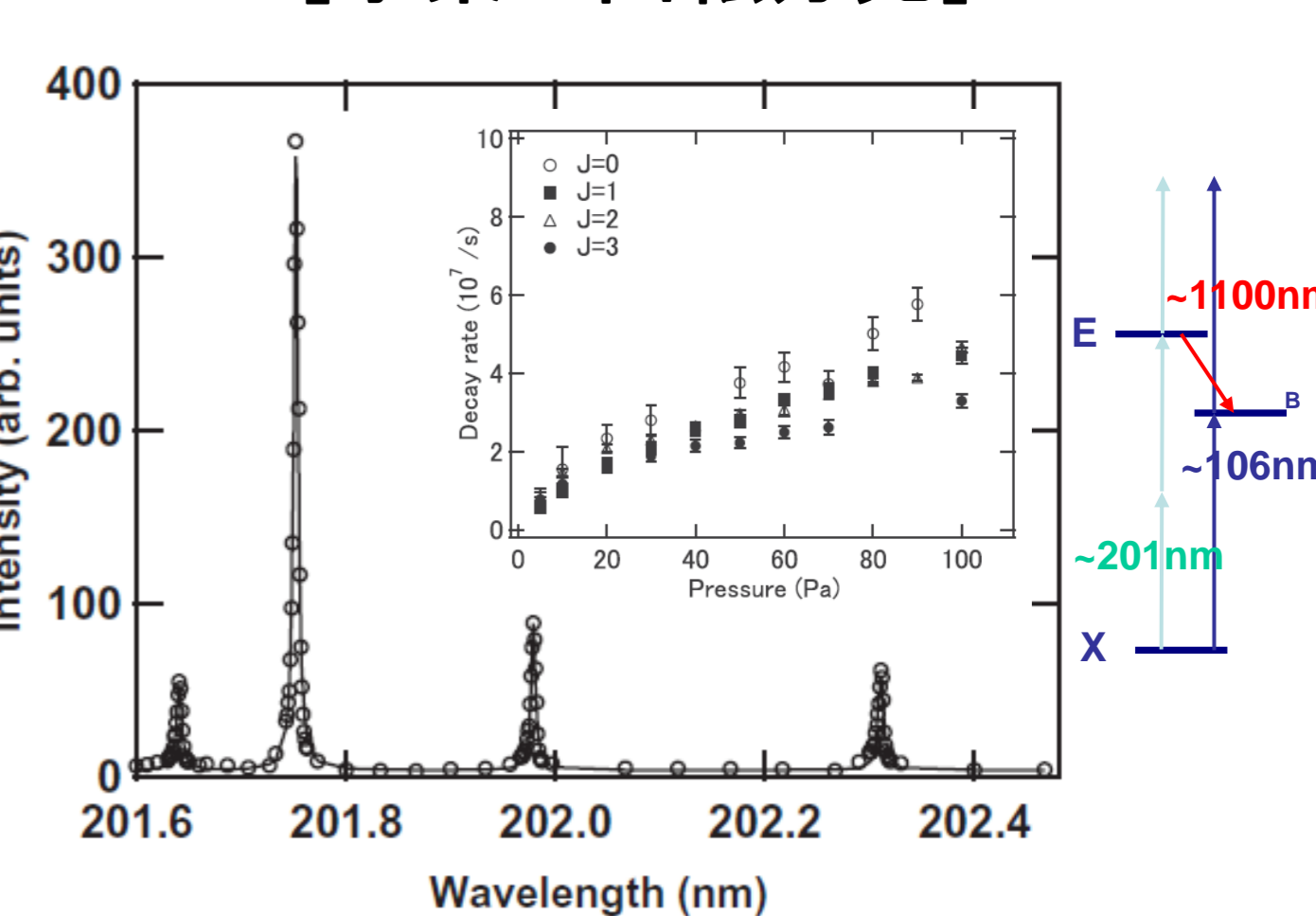
[水素の回転分光]
