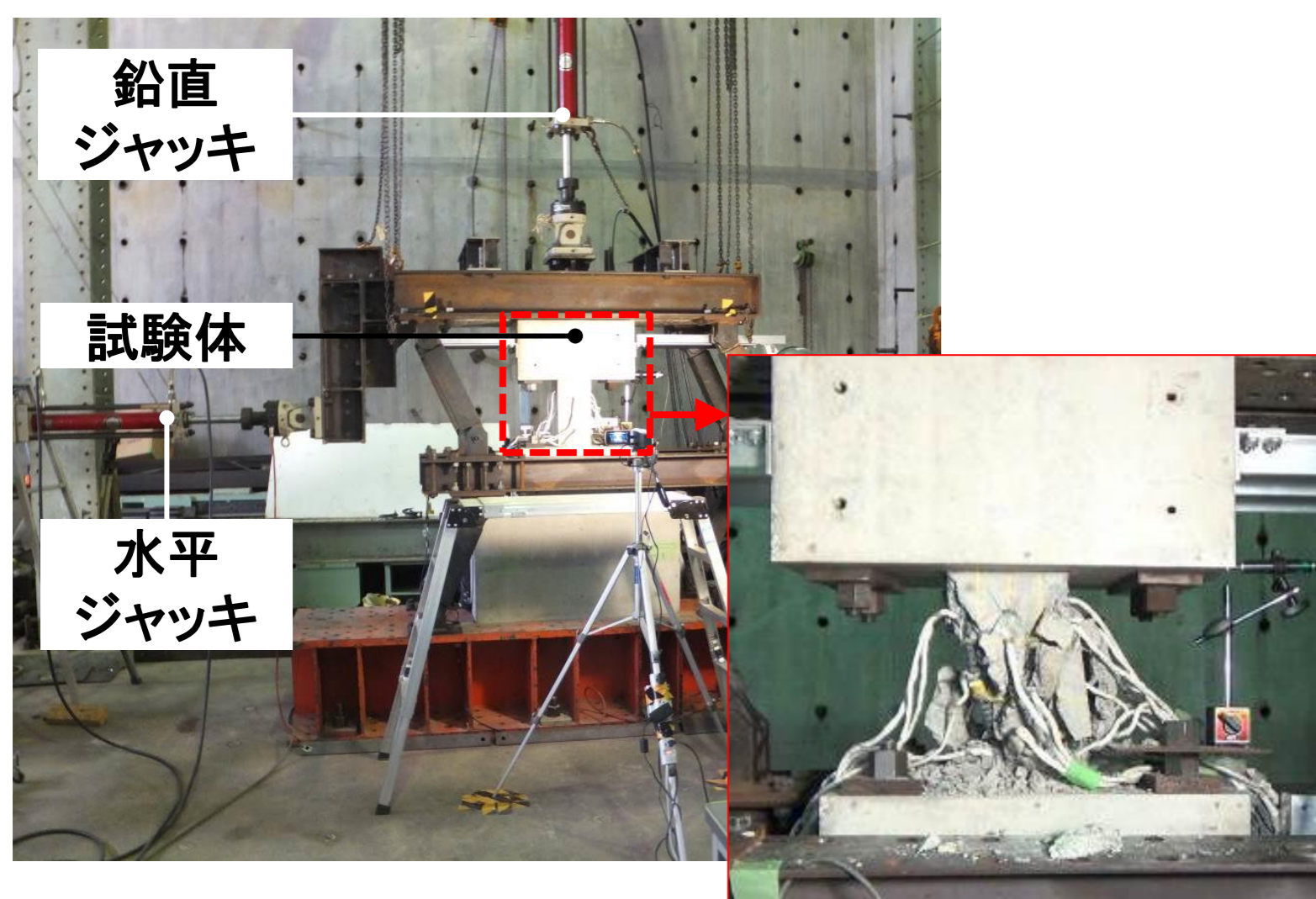
加力装置および軸崩壊後の試験体の様子
