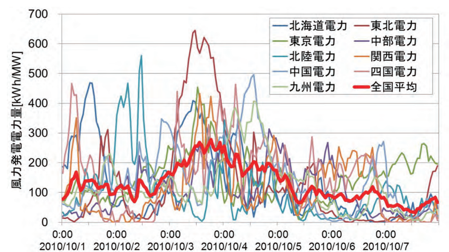
風力発電電力量の変動例
