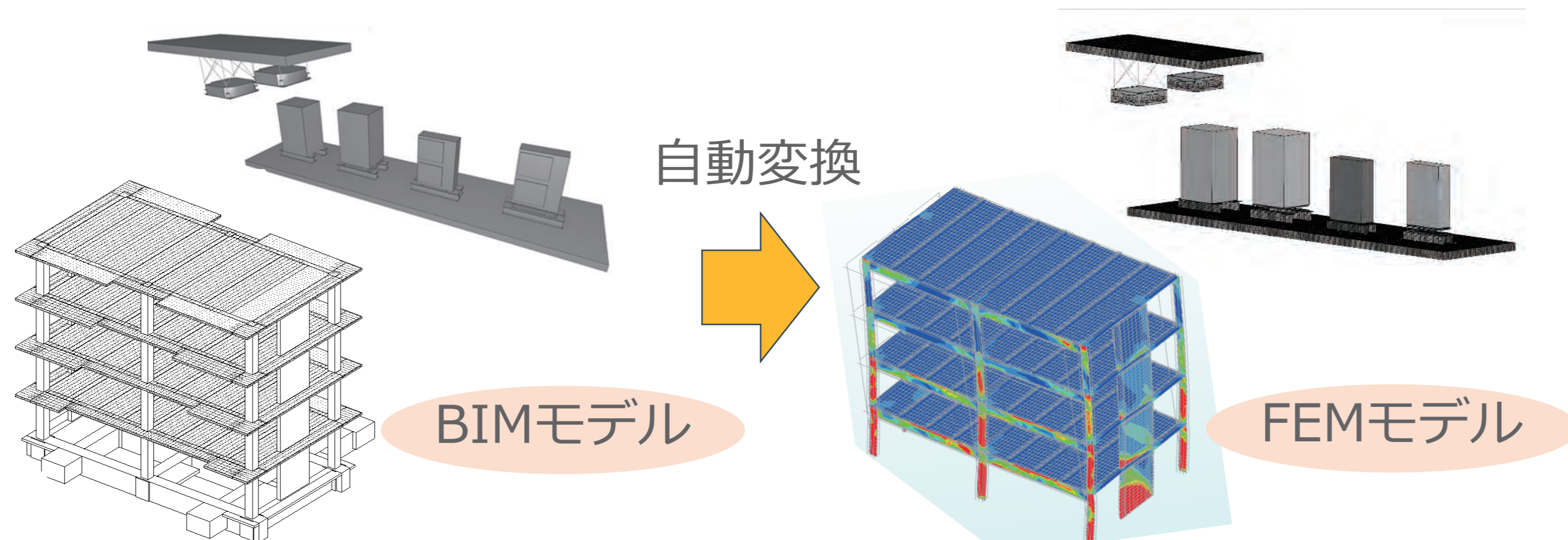
非構造部材を含めたBIM⇒FEM変換システムの開発
