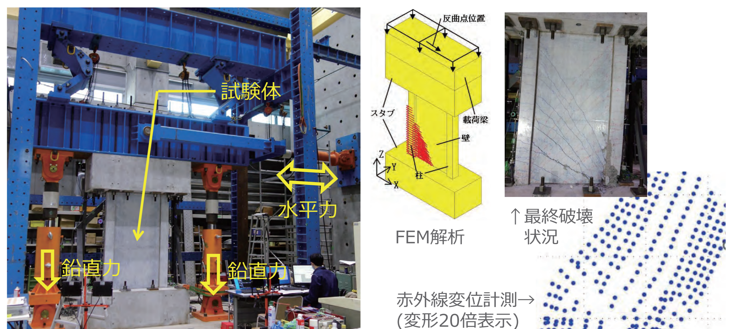
地震時に生じる水平力を模擬した耐震壁の載荷実験
