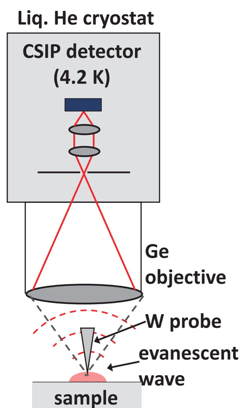
図4. パッシブTHz顕微鏡概念図
