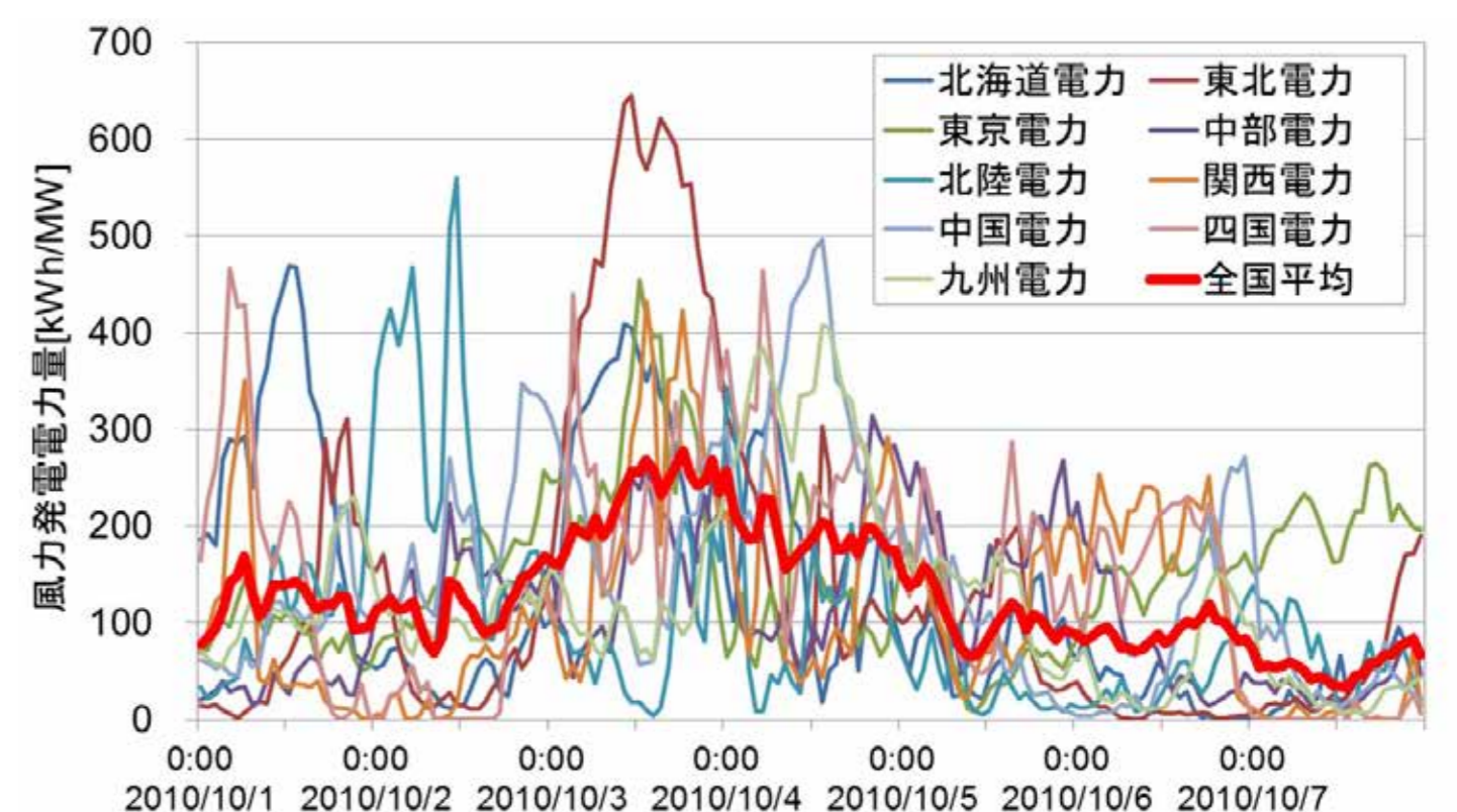
風力発電電力量の変動例
