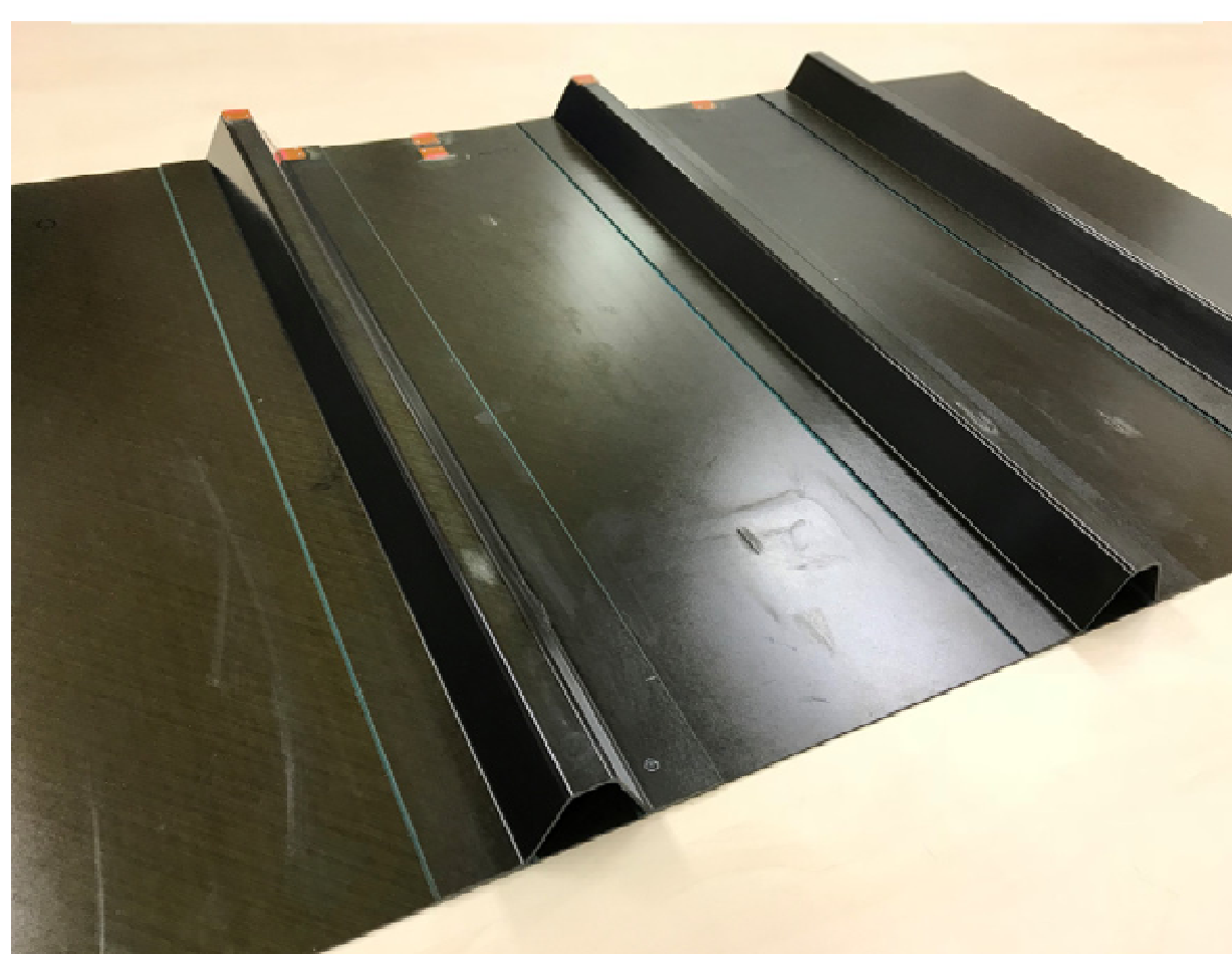
CFRP製補強パネル供試体
