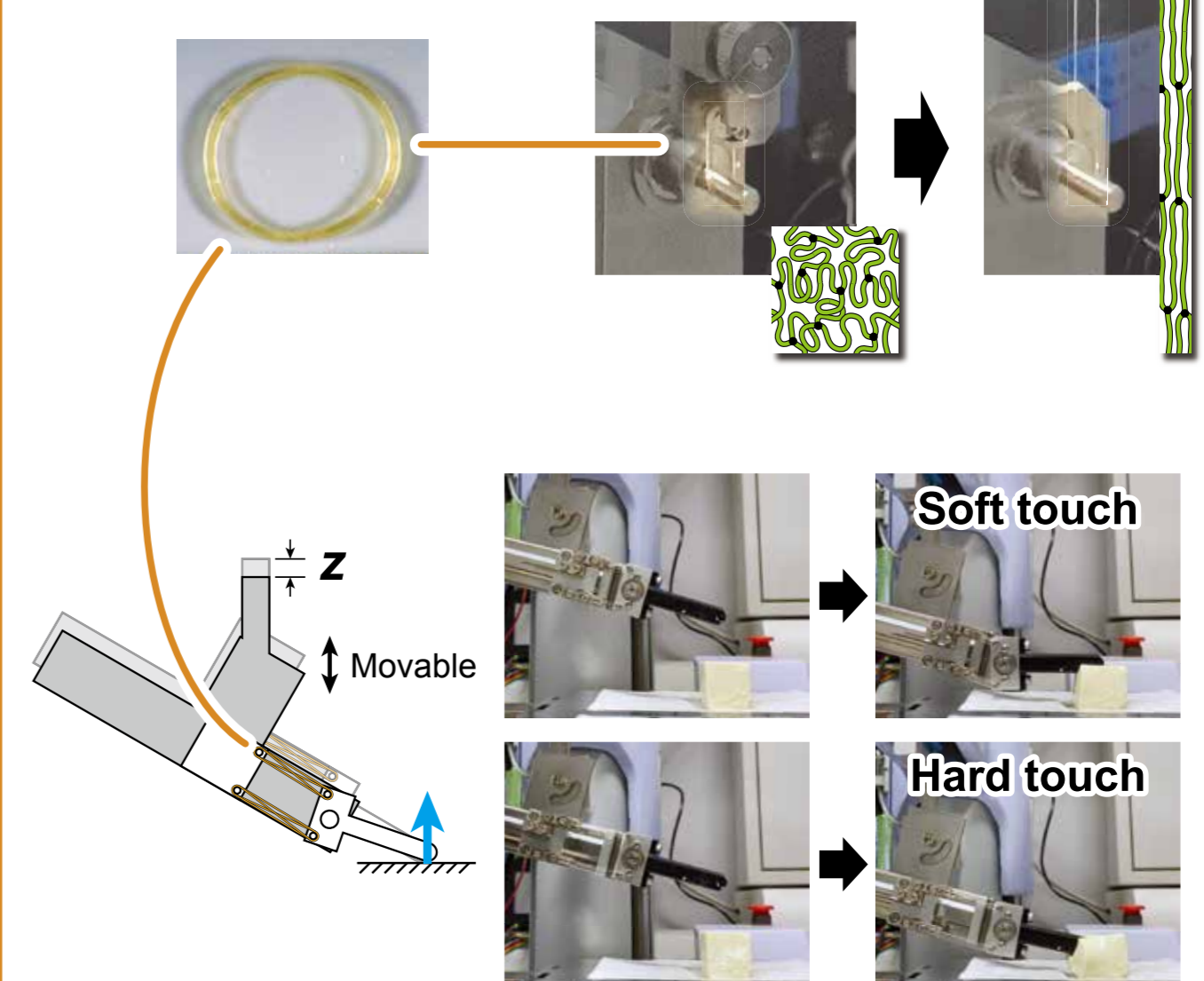
可変剛性アクチュエータへの応用検証実験
