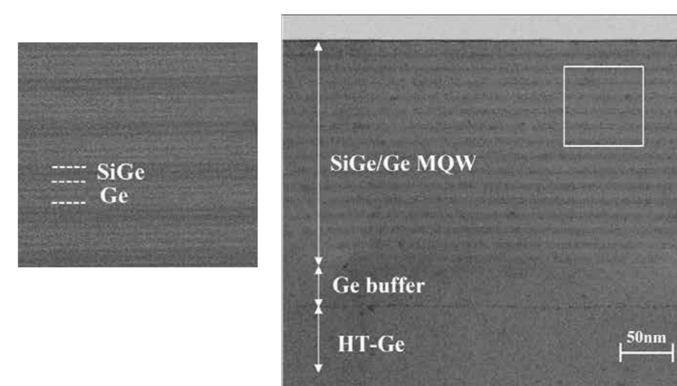
歪みSiGe/Ge多重量子井戸
