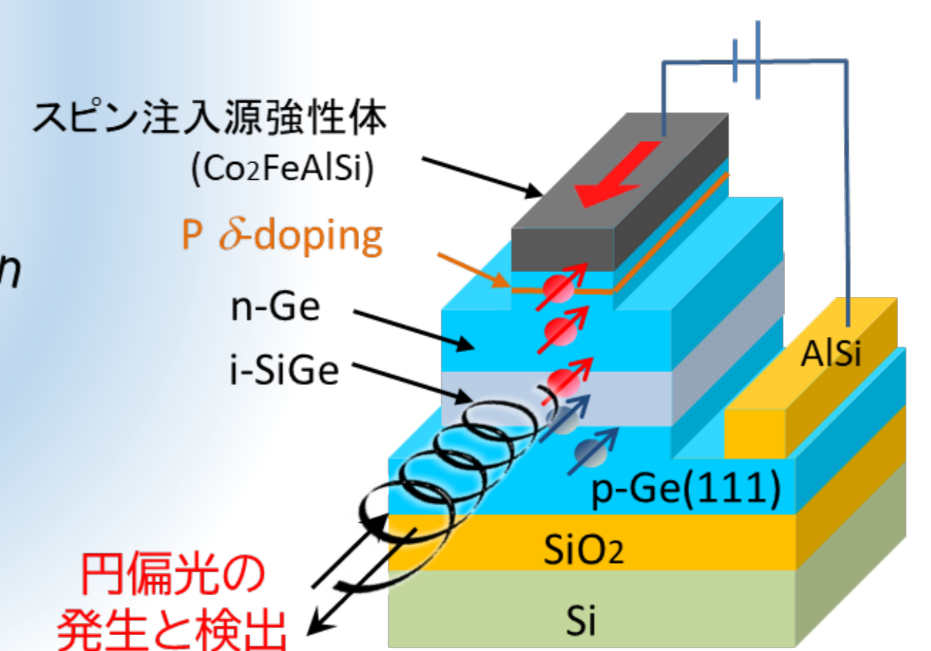
歪みSiGe/GeスピンLED
