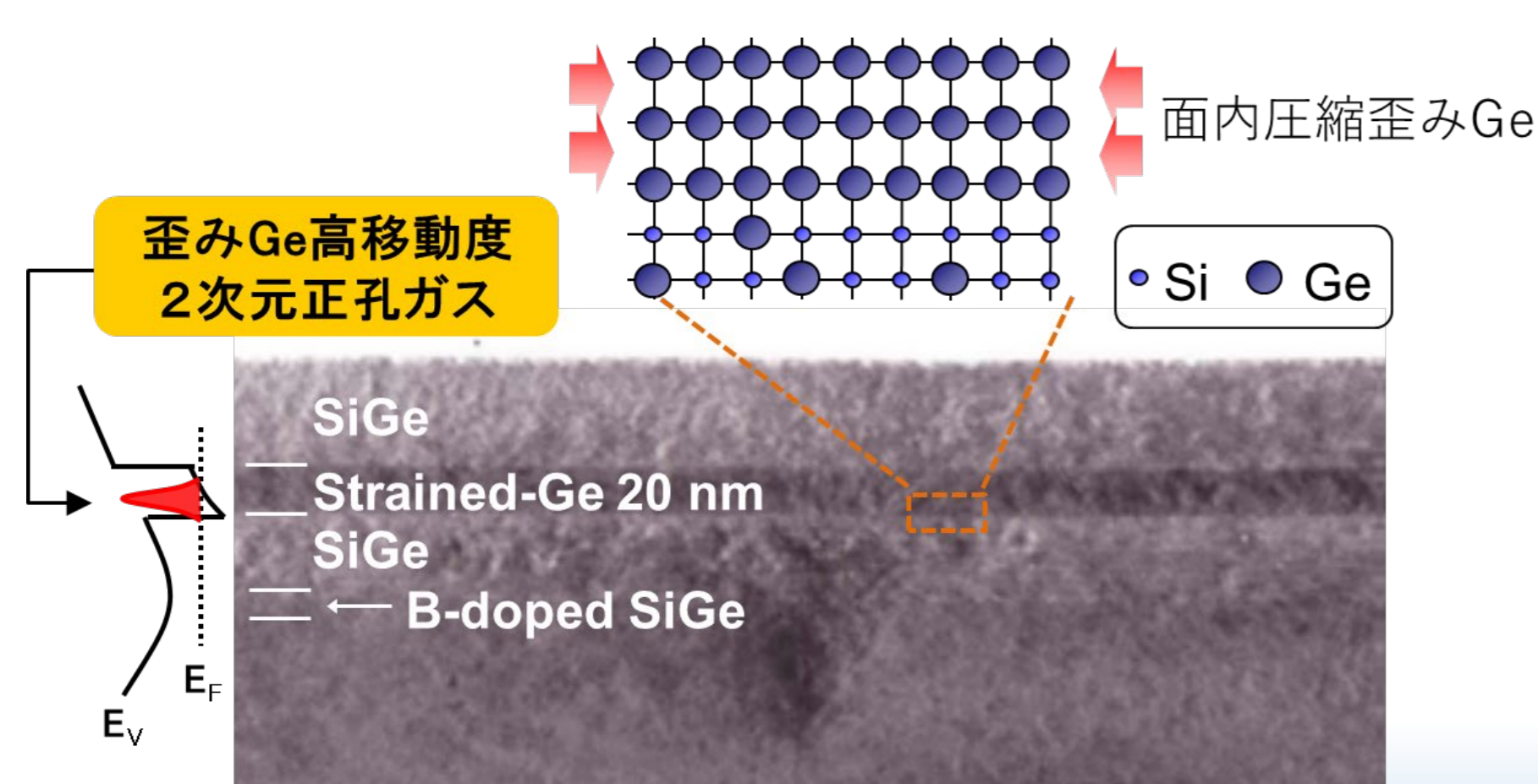
歪みGeチャンネル2次元正孔ガス
