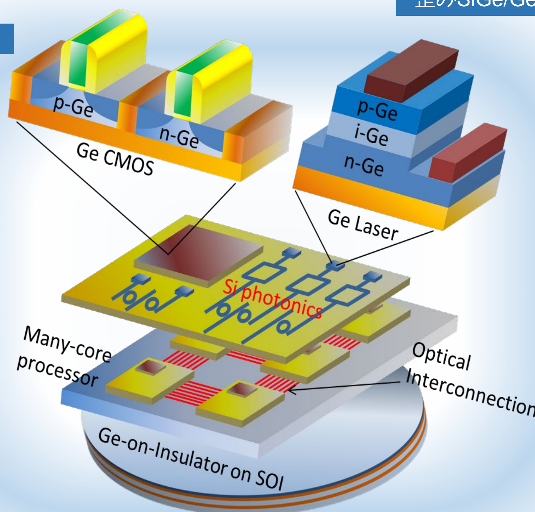
Geプラットフォーム(GOIウェハー)上の光電子融合デバイス集積
