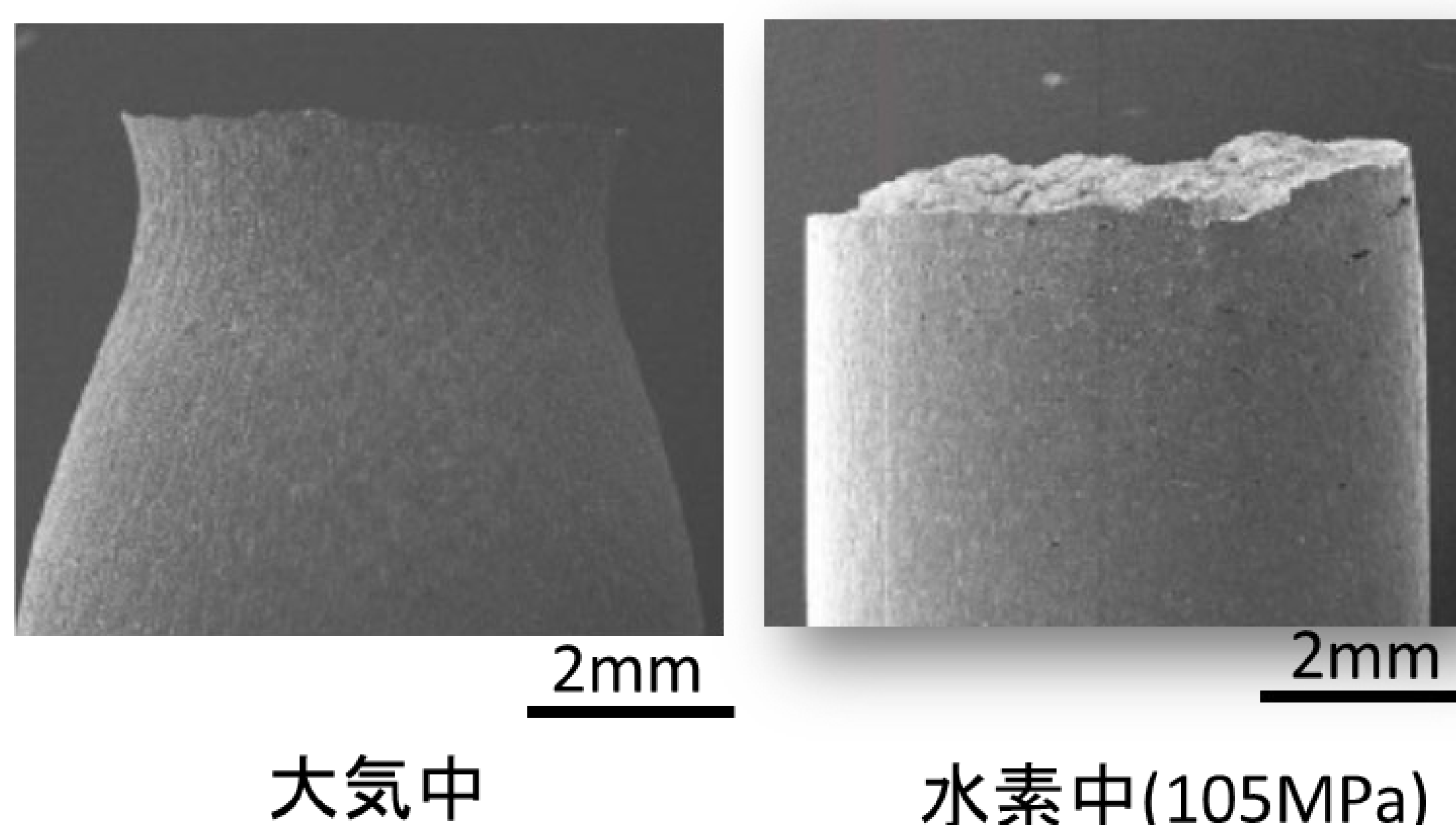
SUS304のSSRT試験後の試験片破断状況
