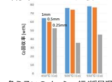
各ふるいのメッシュ幅/緩昇温加熱の違いによるCo回収率の関係
