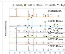
加熱後の正極材のXRDスペクトル
