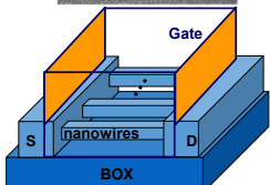
Fig. 1. 次世代デバイス構造と期待されるシリコンナノワイヤトランジスタを試作し電気伝導特性を解明。
