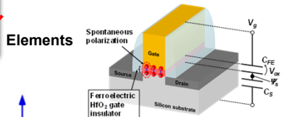
Fig. 6. 物理限界を突破して急峻なサブスレシールド特性を実現する負性容量トランジスタ技術。
