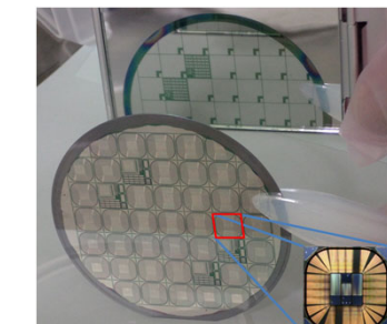
Fig. 2. IGBTと呼ばれるシリコンパワーデバイスの研究に着手。スケールリング(微細化)により耐圧3300Vを達成することに、ダブルゲートIGBTによる損失低減にも成功。
