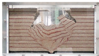
室内模型実験による、土砂流出、空洞生成・拡大、陥没メカニズムの再現
