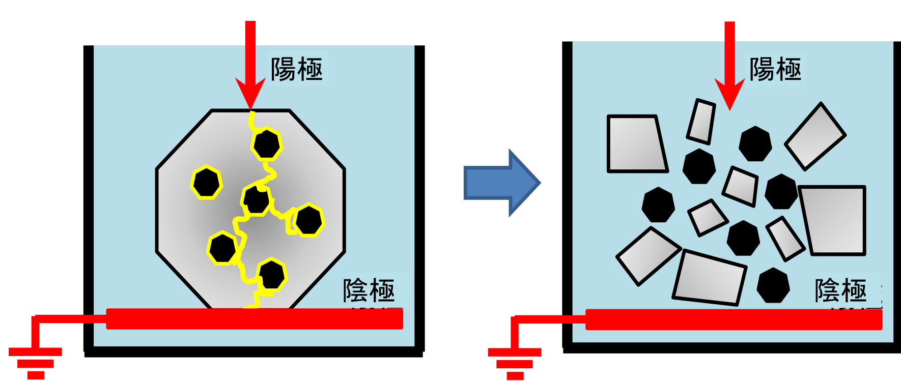
電気パルス粉碎の破壊概念図
