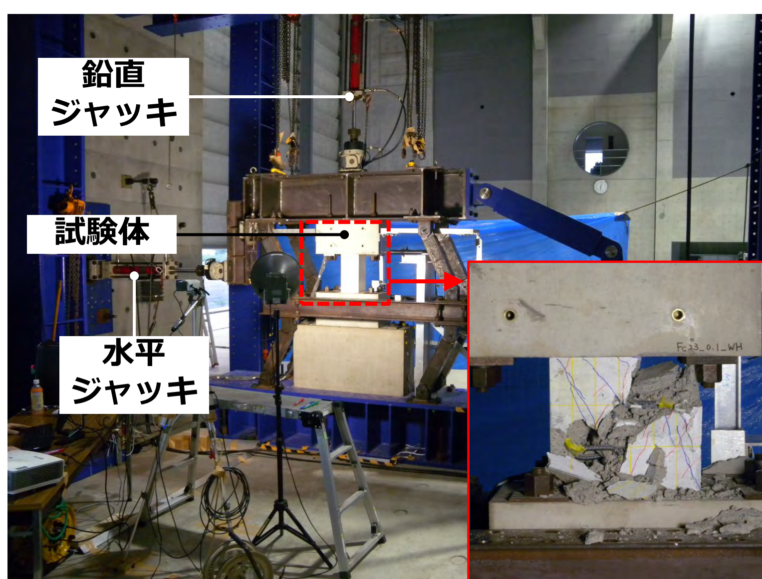
加力装置および軸崩壊後の試験体の様子
