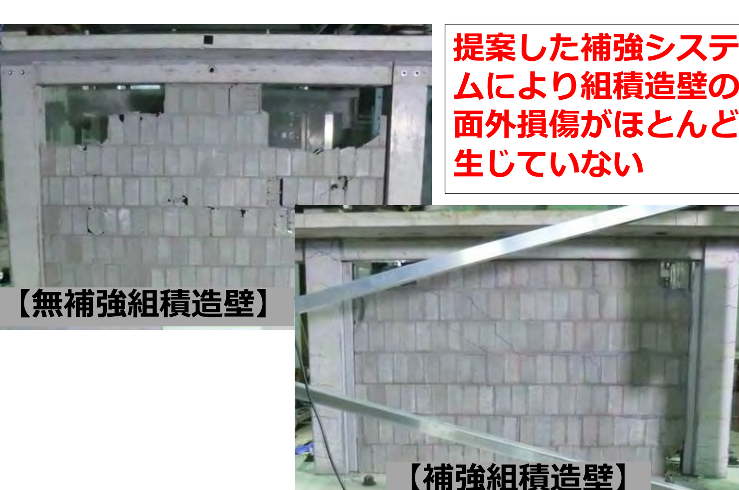
無補強および補強組積造壁の損傷状況
