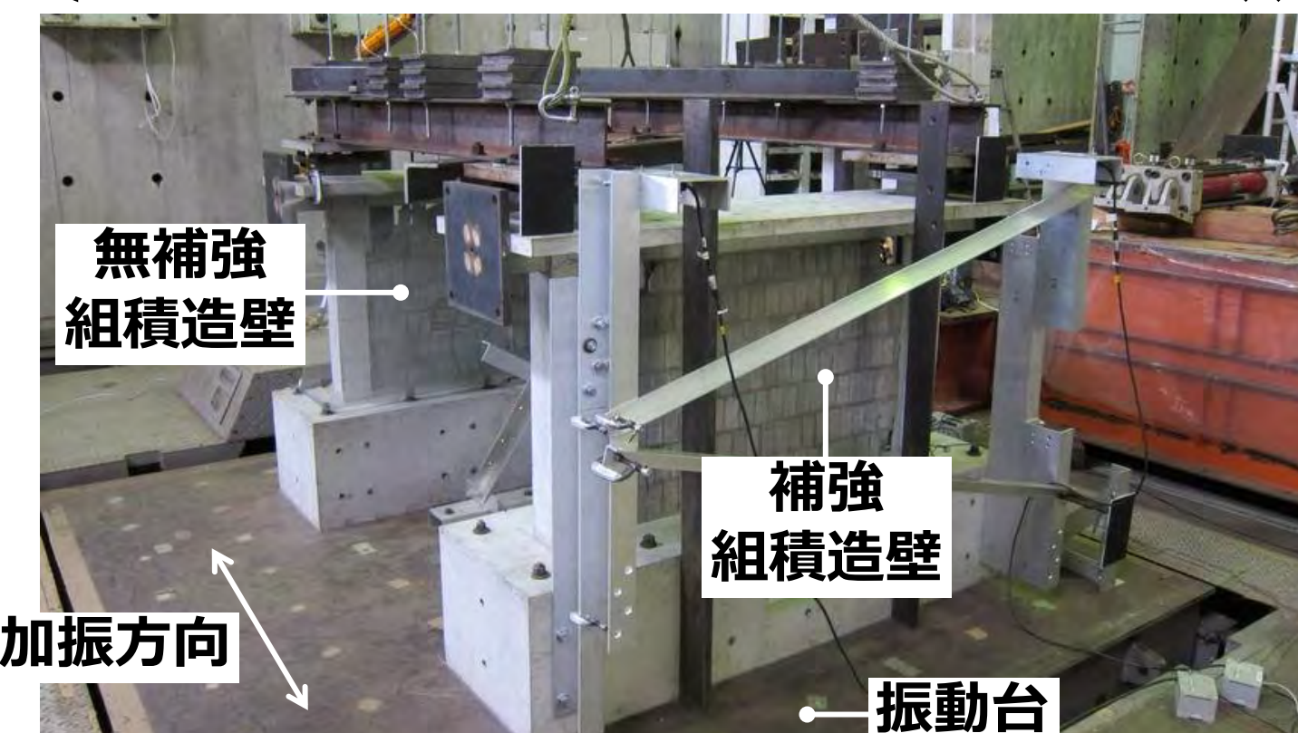
振動台実験の様子および入力標準加速度波形
