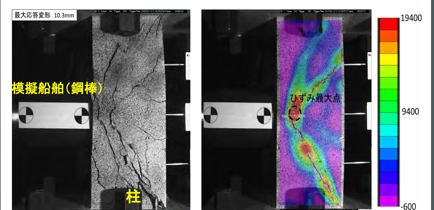
鉄筋コンクリート造柱への模擬船舶の衝突実験
