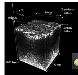
堆積層内3次元音響画像
