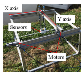
音響コアリングシステム
