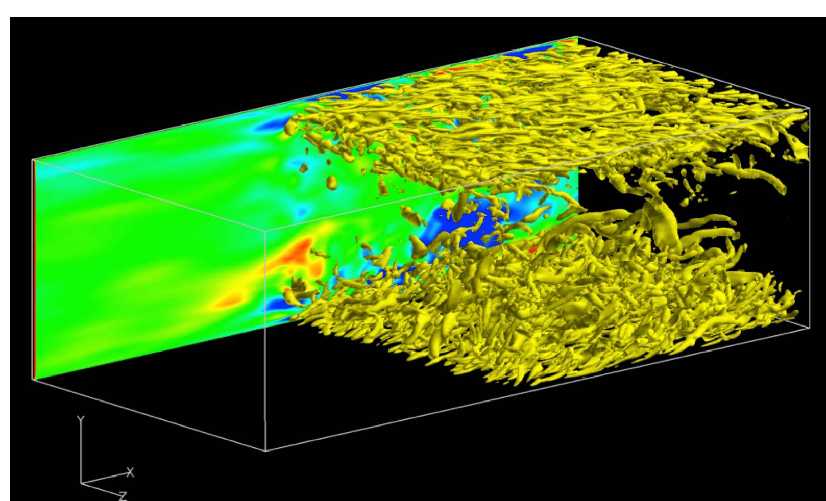
図1 チャンネル乱流の壁近くの渦
