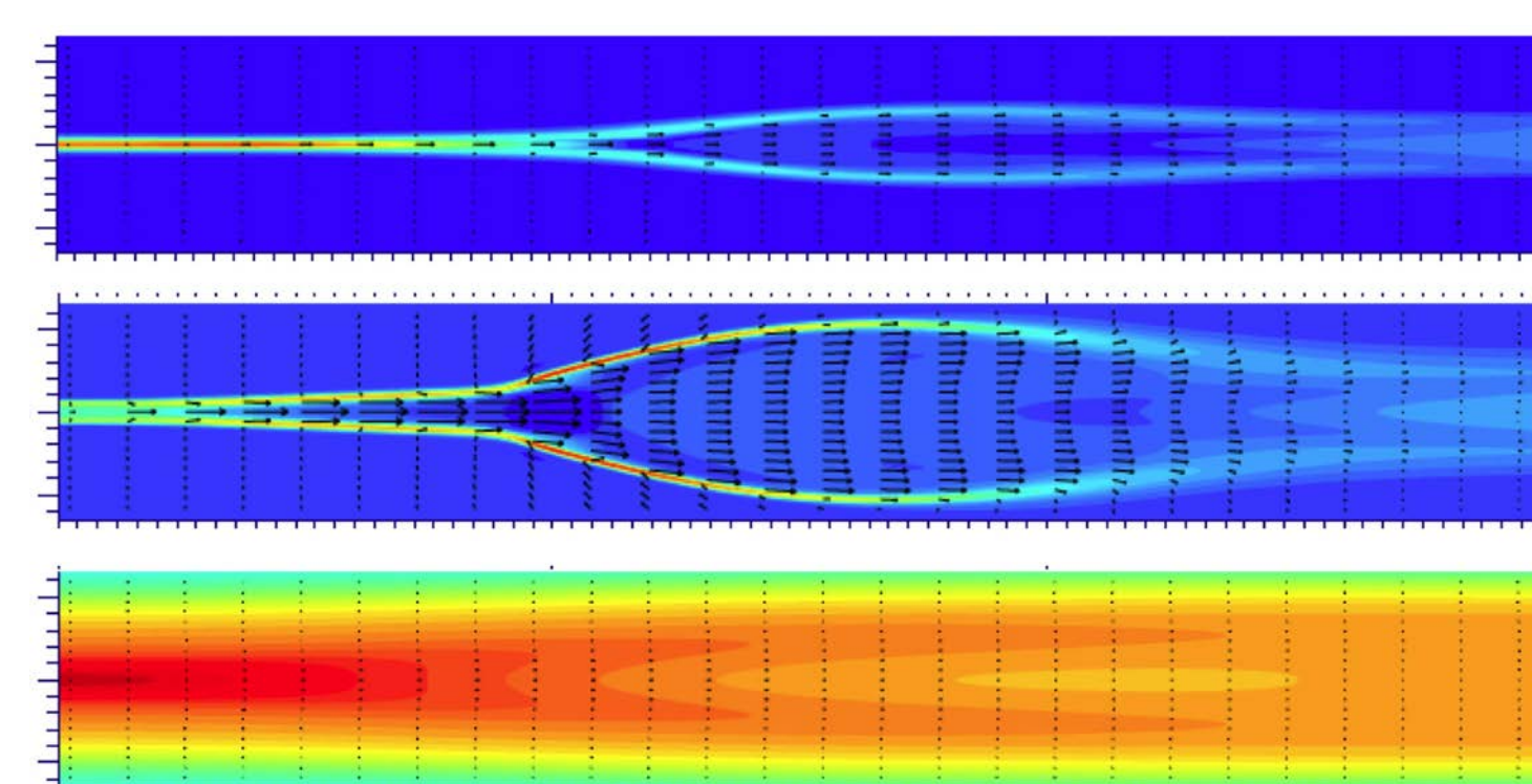
図3 磁気リコネクションのジェット
