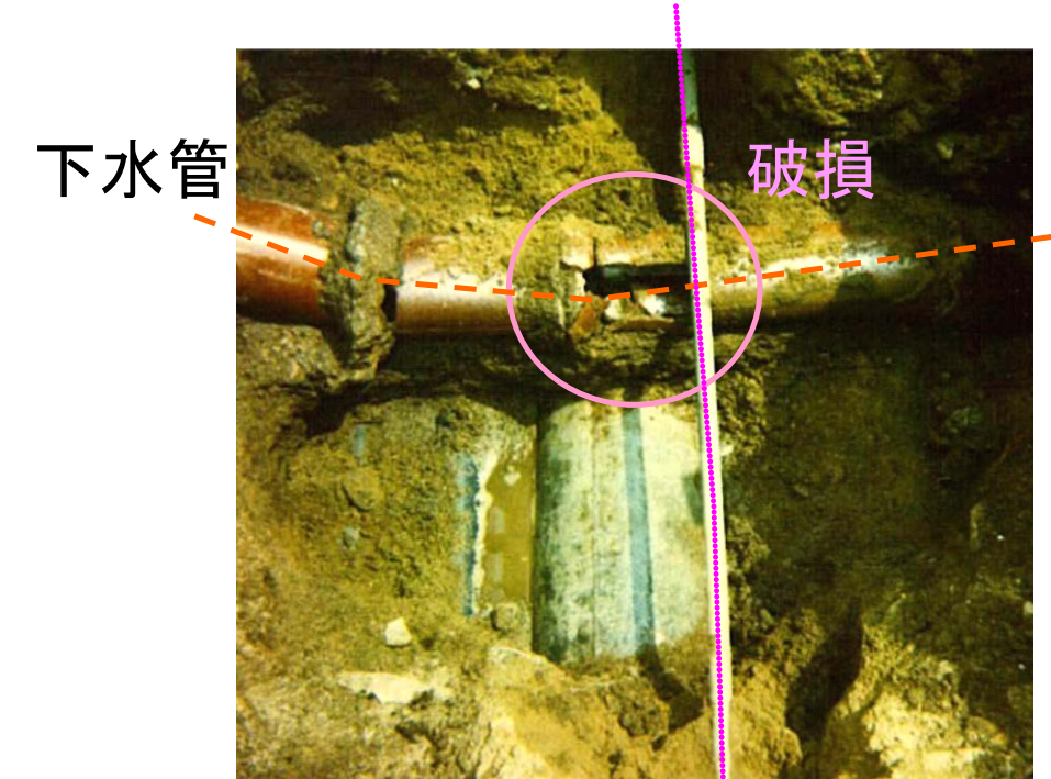
錯綜する地中埋設物と下水管の破損
