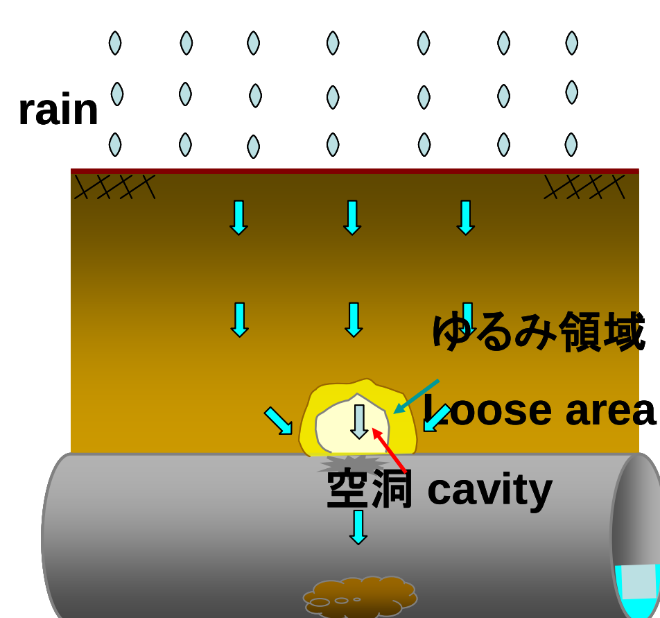
埋設管破損による土砂流出と空洞形成
