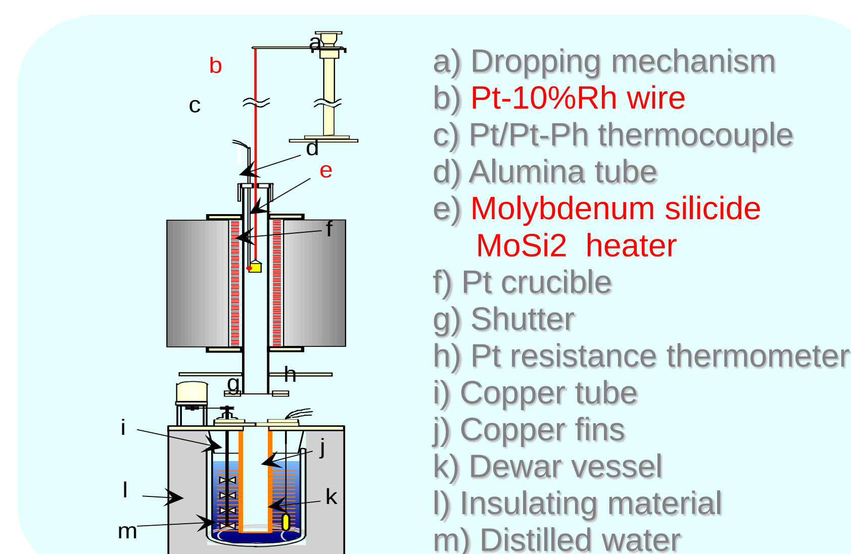
図4. 1600℃まで使用可能な高温落下型熱量計
