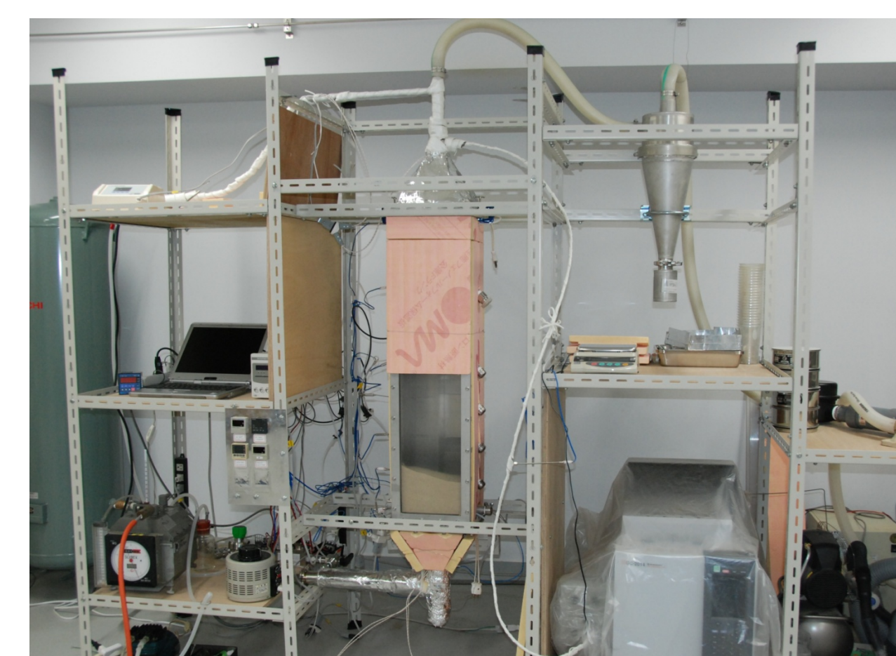
乾燥試験装置
