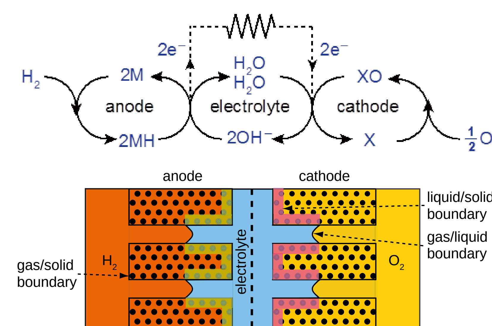
燃料電池/電池(FCB)の作動原理
