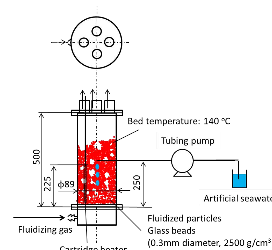
流動層蒸発実験装置
