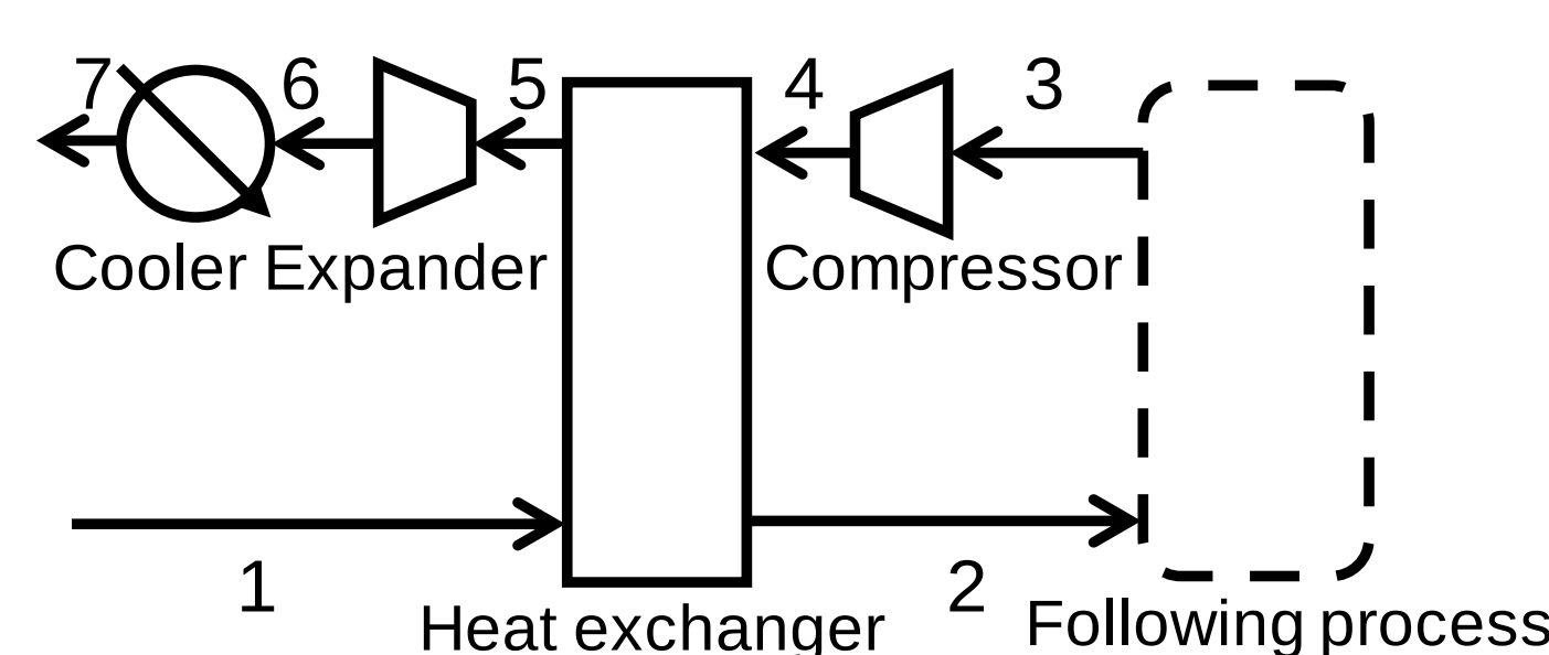
自己熱再生プロセスフローダイアグラム (プロセス流体: 気体)
