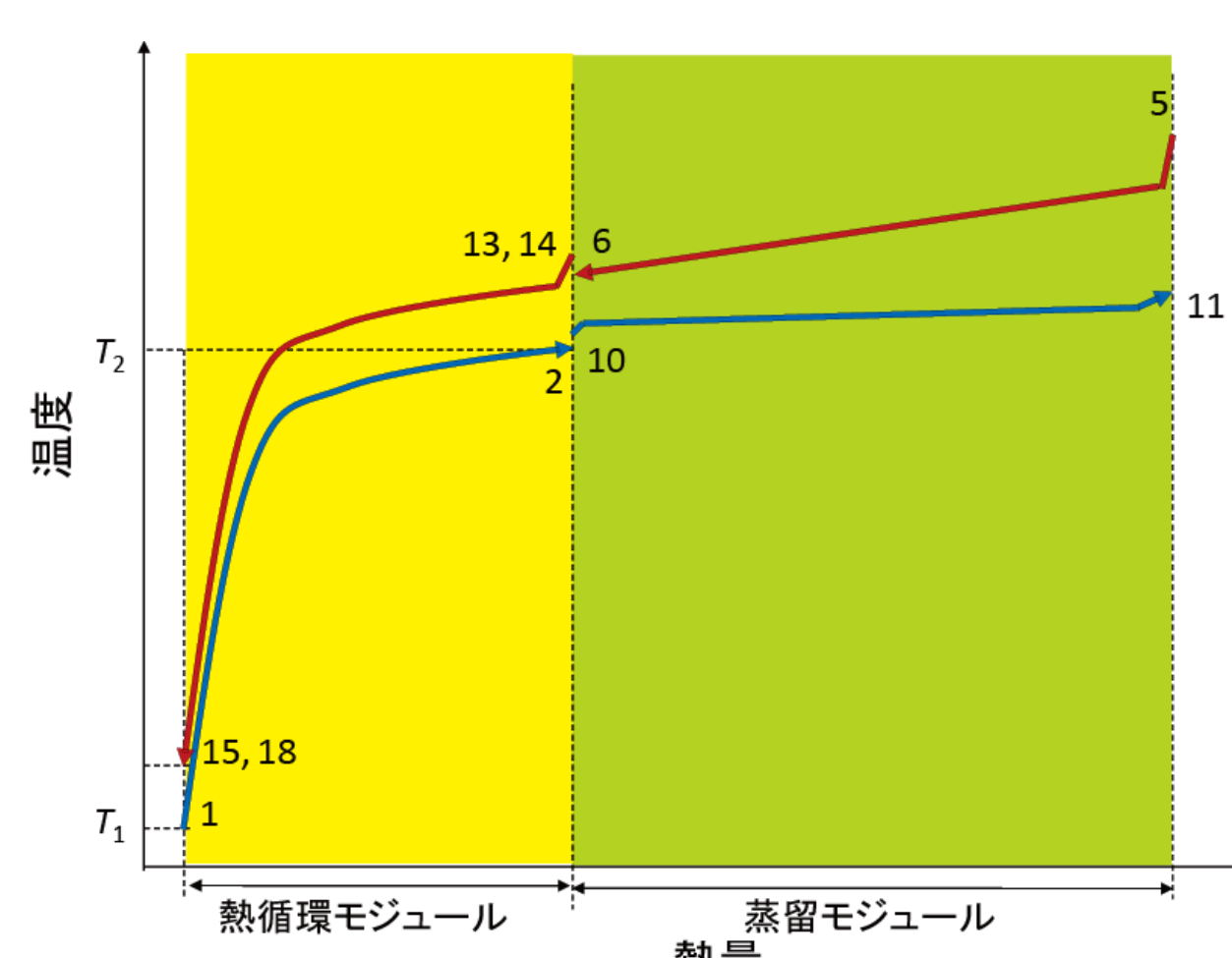
自己熱再生蒸留温度-熱量線図
