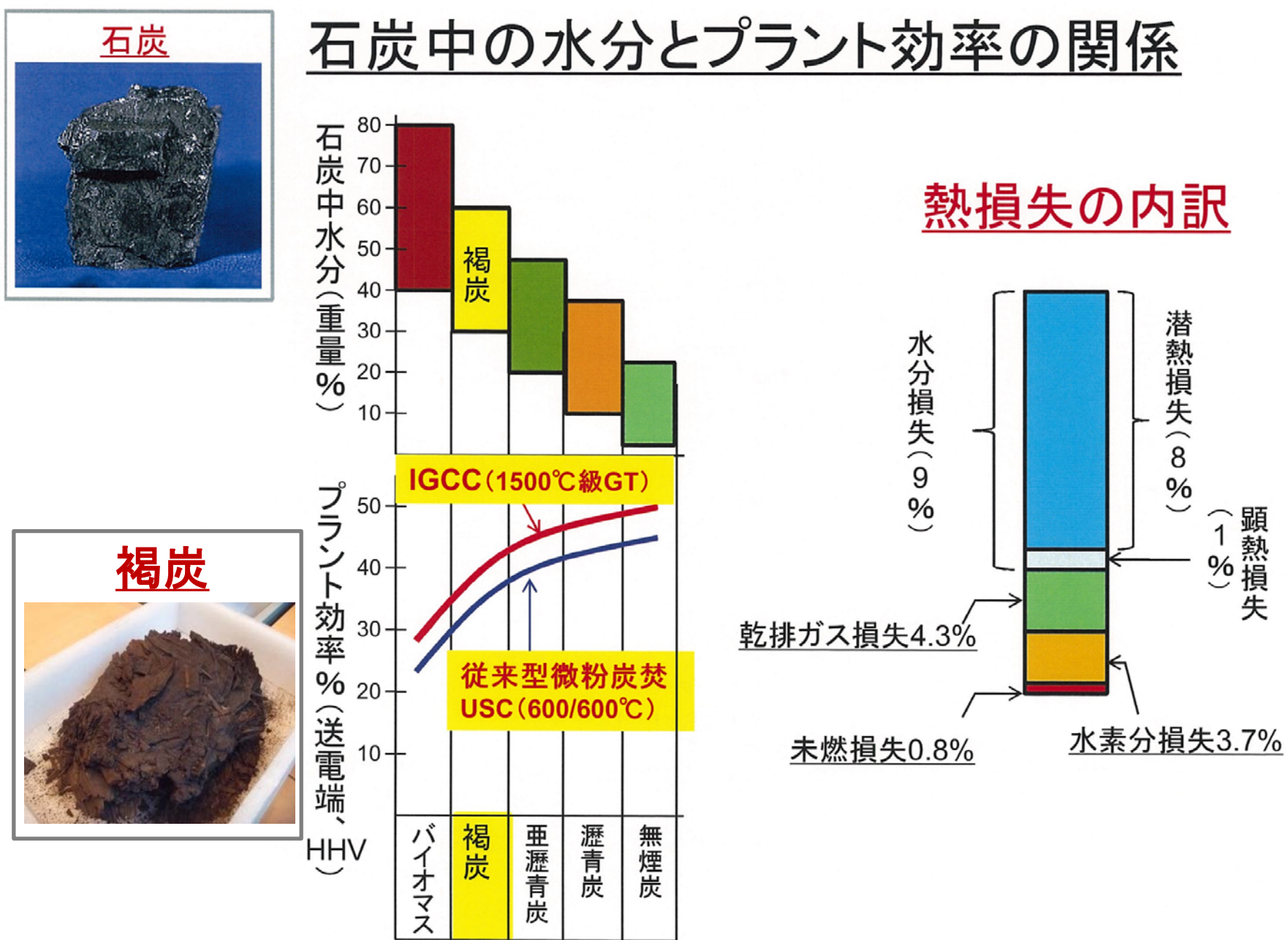
石炭の種類と熱効率
