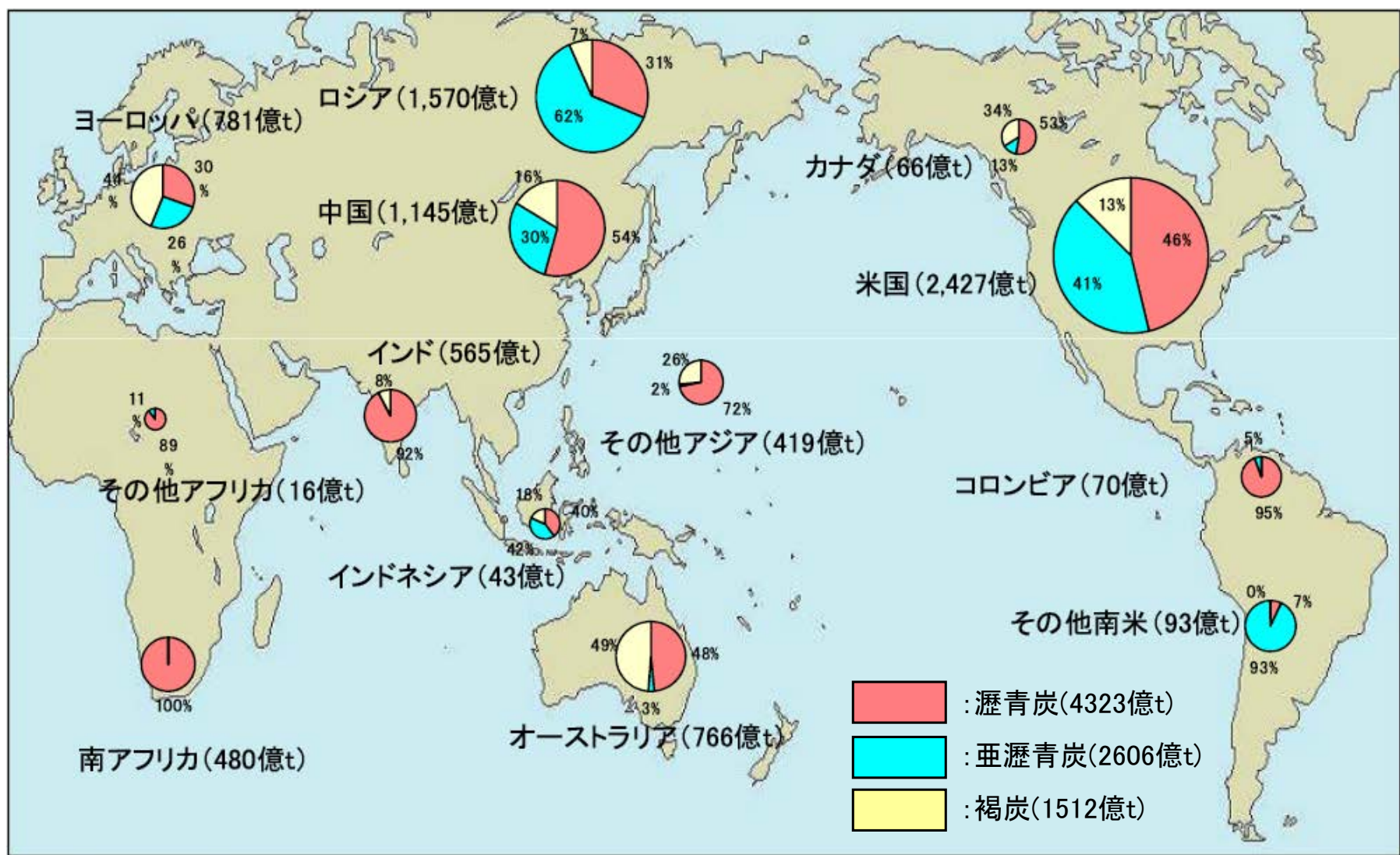
世界の石炭資源
