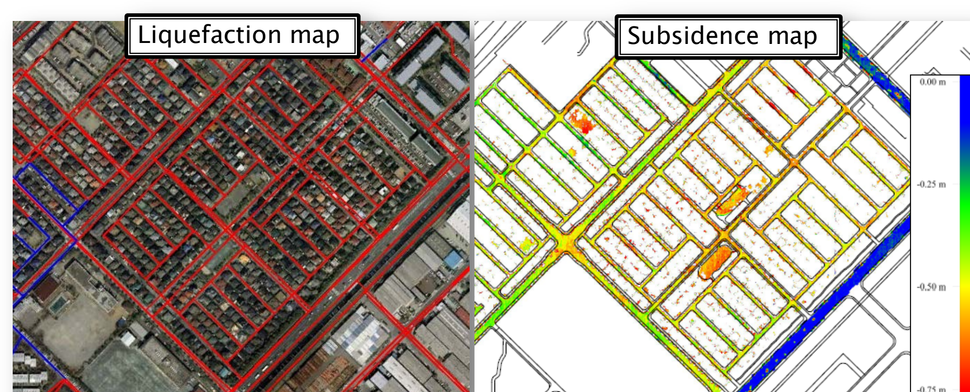
航空レーザによる液状化地盤沈下マップ
