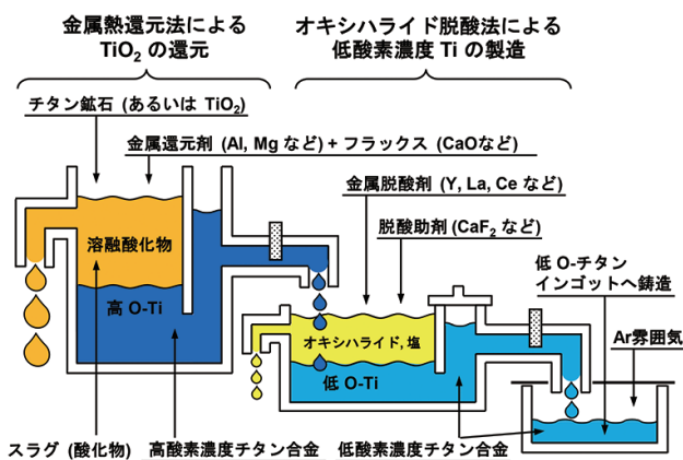
図 イットリウム (Y) などのオキシハライド (YOF など) の生成反応を応用して、高酸素濃度のチタン合金から酸素を直接、除去する新製錬法の概念図。アルミニウムのスクラップなどを利用することにより、CO 2 の発生量を大幅に低減できる新規製錬プロセスの構築が可能。
